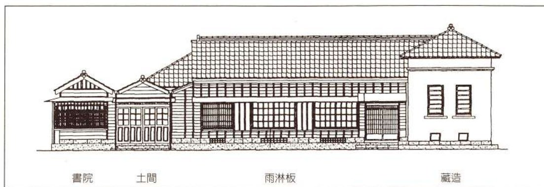
建築立面圖示 漢光建築師事務所提供
